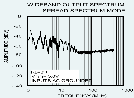
IU8632E扩频技术频谱能量图
