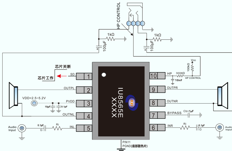
应用线路图
