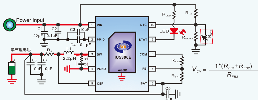
IU5306E外部设定浮充电压应用电路图
