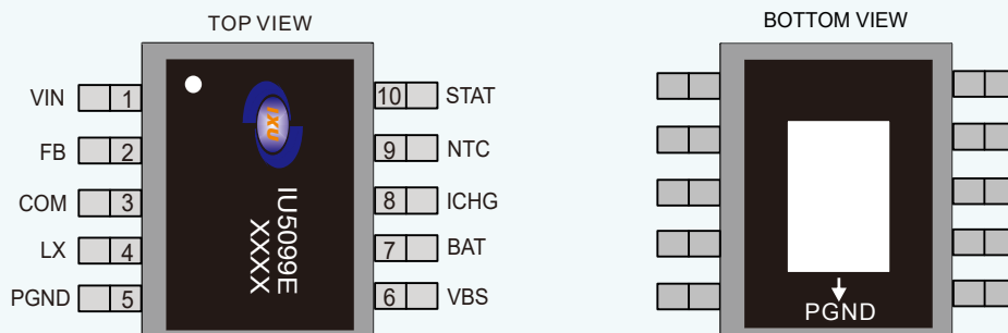
e-MSOP10 IU5099E
