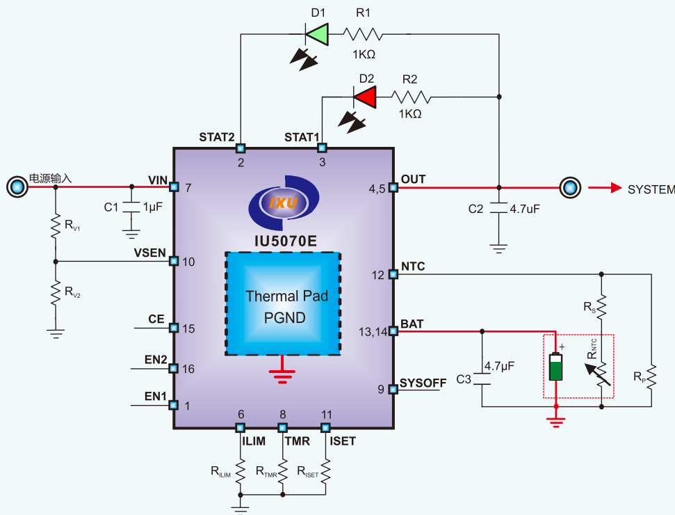
IU5070E应用电路图
