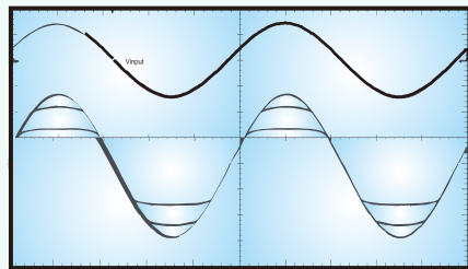
CS8736E功率限制波形
