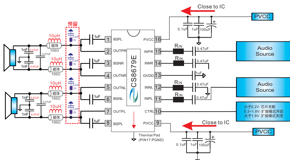
图1 单端输入立体声输出典型应用图
