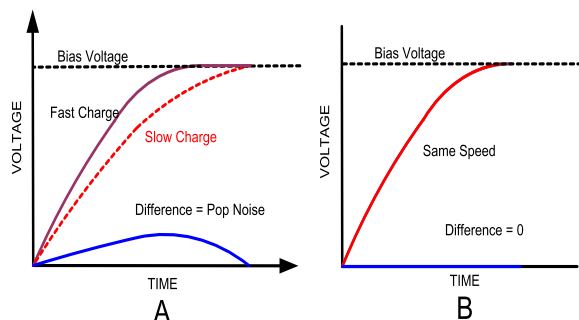
图5 差分输入偏置电压建立过程
