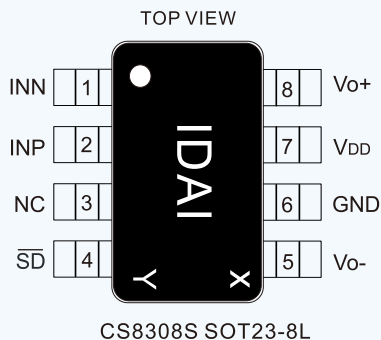
CS8308S SOT23-8L
