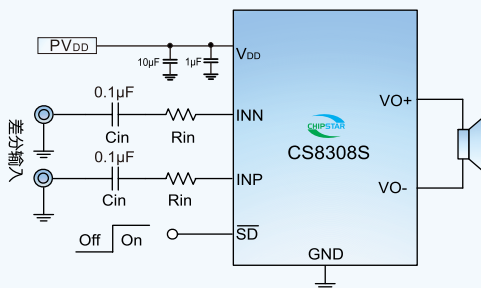
图1 CS8308S差分输入方式应用图
