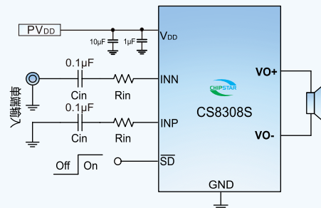
图2 CS8308S单端输入方式应用图
