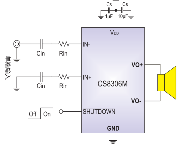
图2 CS8306M单端输入方式应用图
