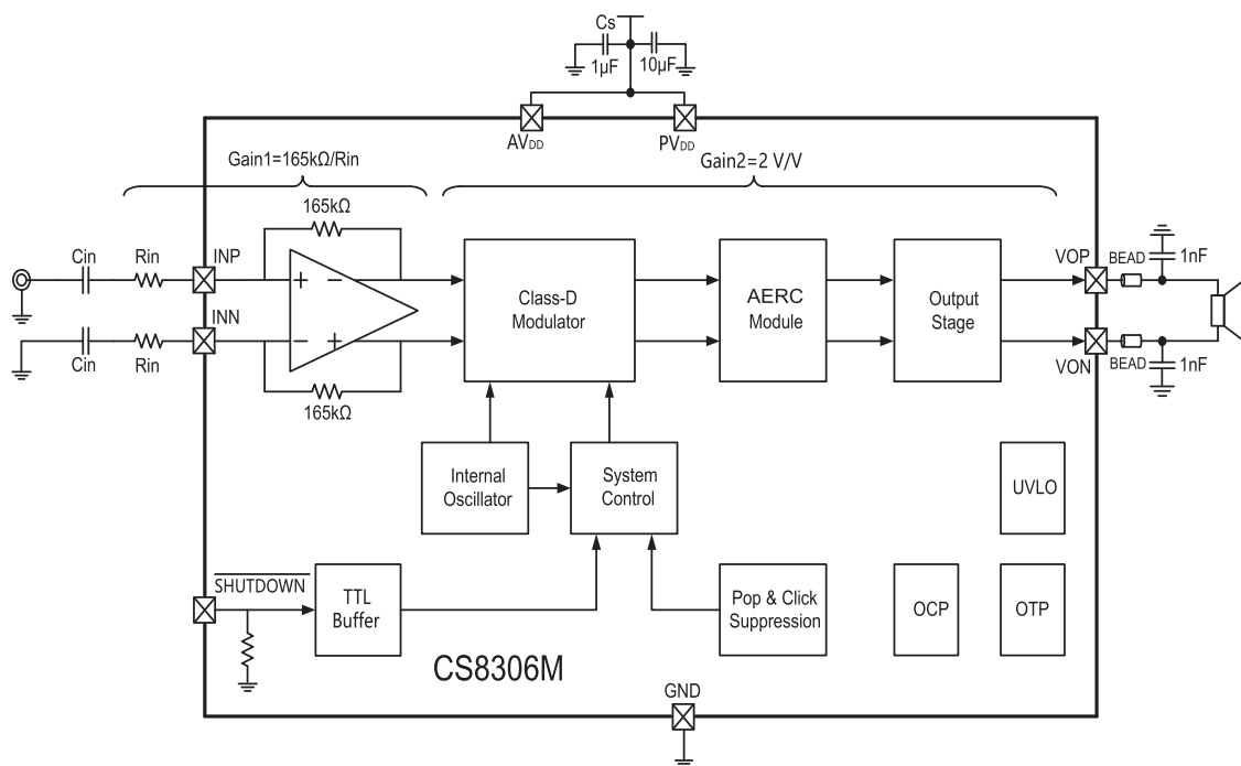
CS8306M功能框图
