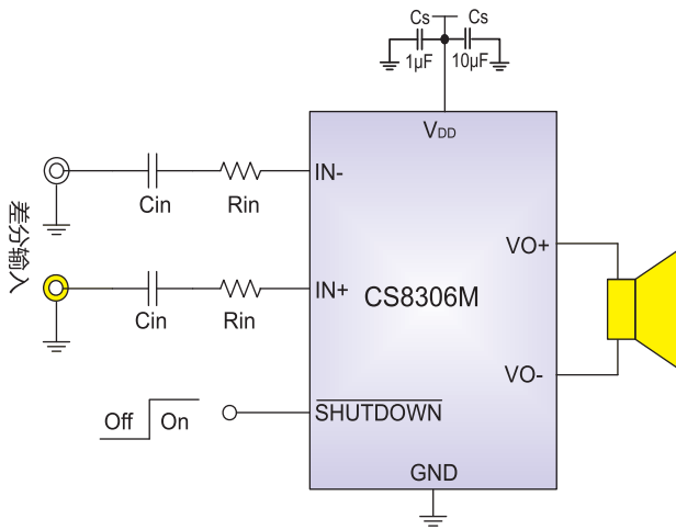
图1 CS8306M差分输入方式应用图
