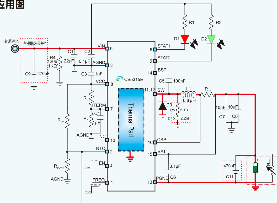
CS5315E应用电路图
