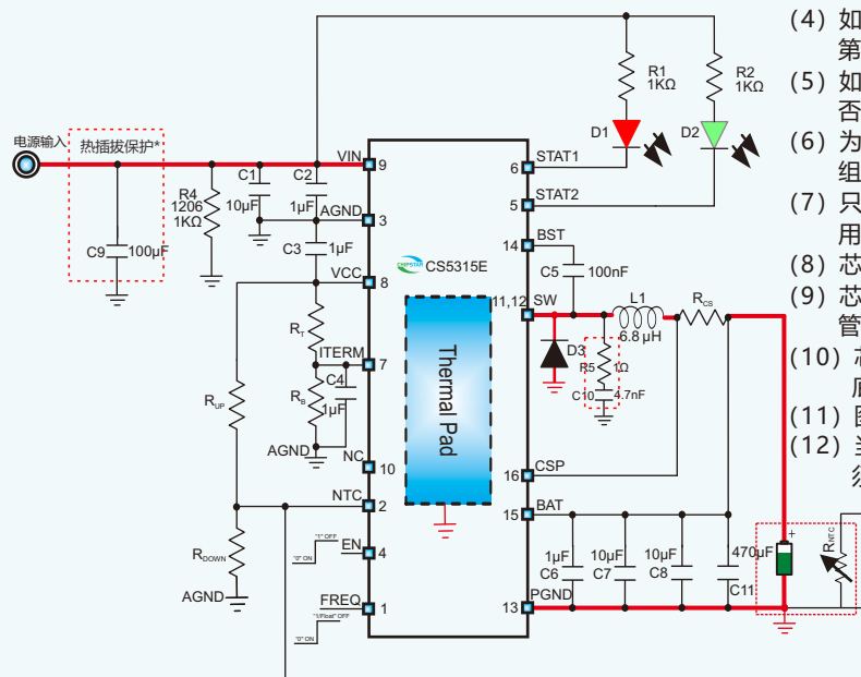
CS5315E应用电路图
