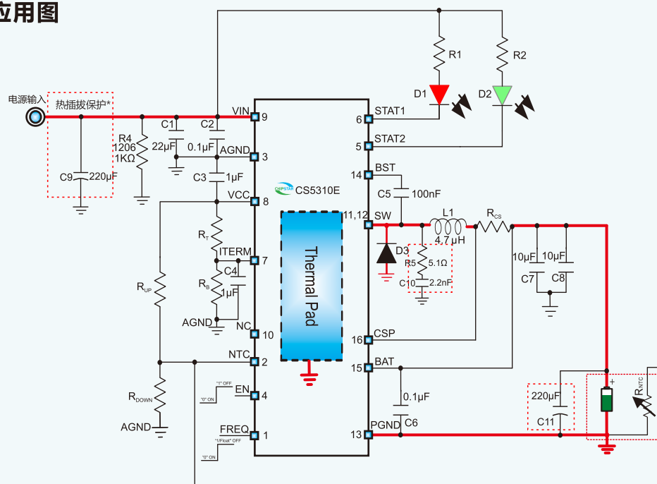
CS5310E应用电路图
