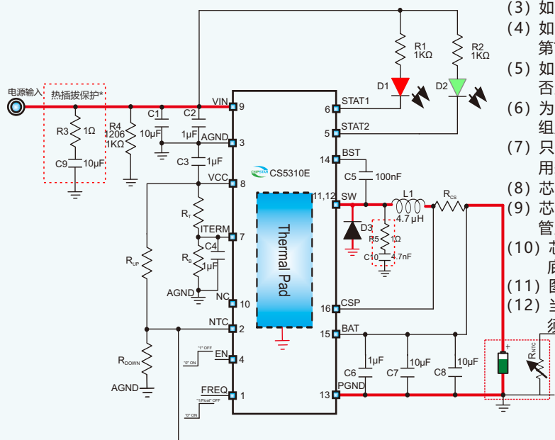
CS5310E应用电路图
