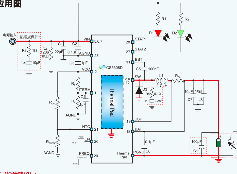
CS5308D应用电路图
