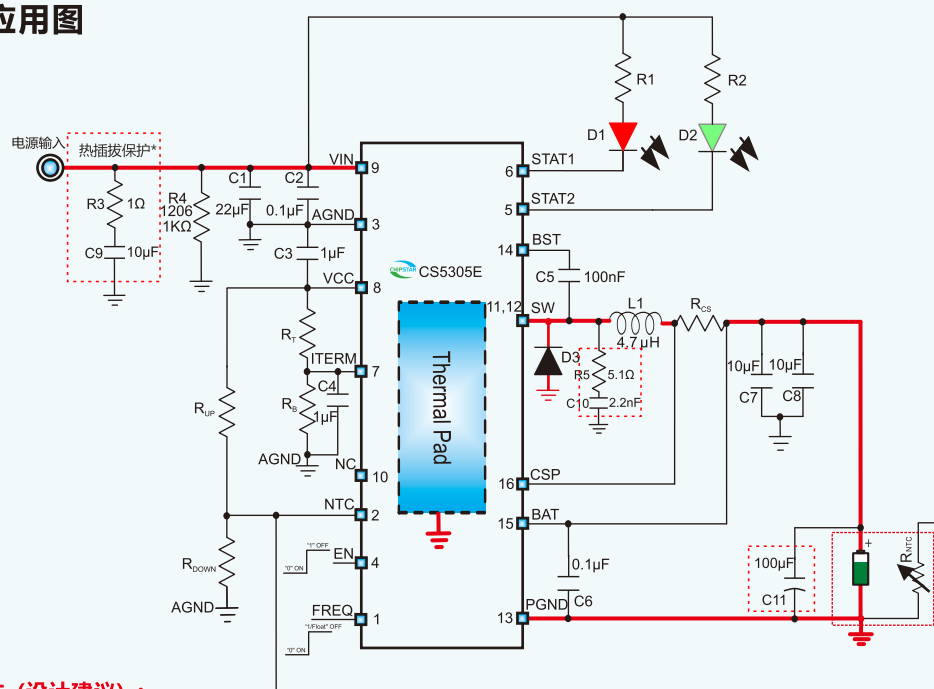
CS5305E应用电路图
