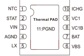
DFN3X3_10L CS5086D
