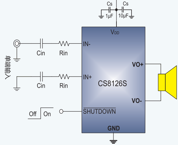
图2 CS8126S单端输入方式应用图
