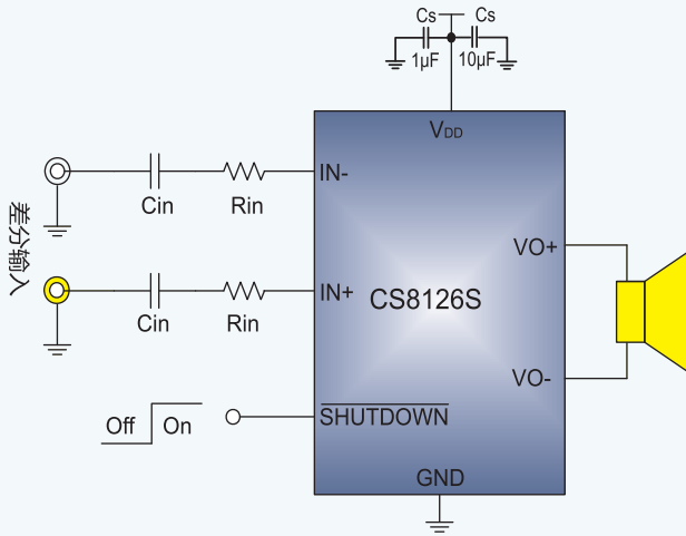
图1 CS8126S差分输入方式应用图
